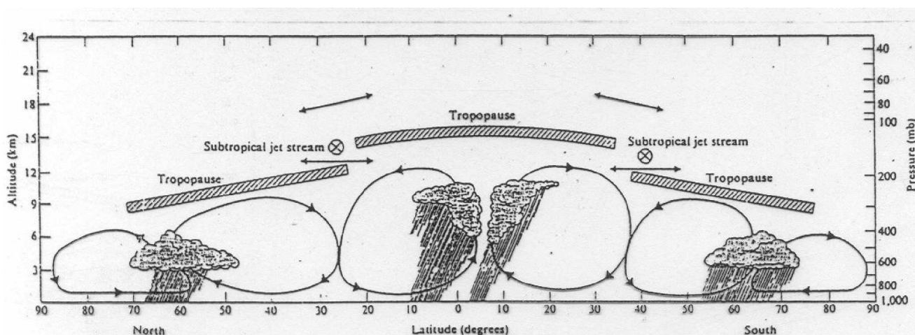
Figura 5.14 - Representação esquemática da circulação global na troposfera durante o verão (Hemisfério Norte).
